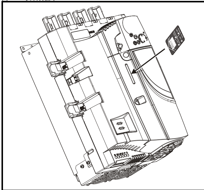
图 9-1 安装智能卡
