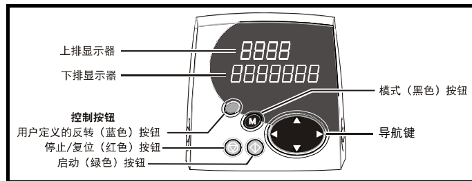
图 5-1 SM-键盘
