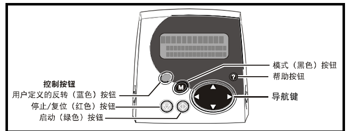
图 5-2 MP-键盘
