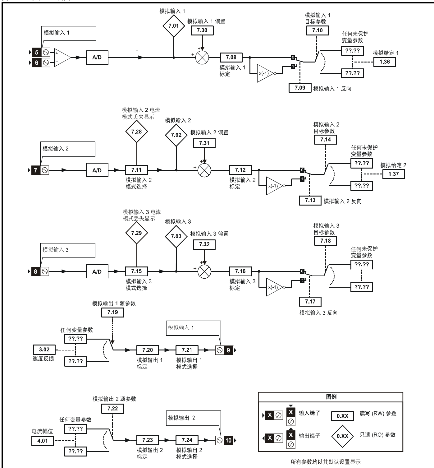
图 11-8 菜单 7 逻辑图
