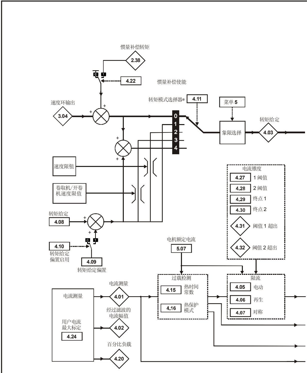
图 11-4 菜单 4 逻辑图
