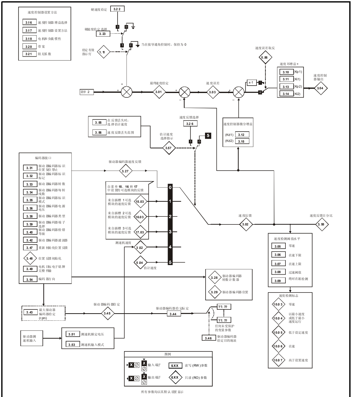
图 11-3 菜单 3 逻辑图
