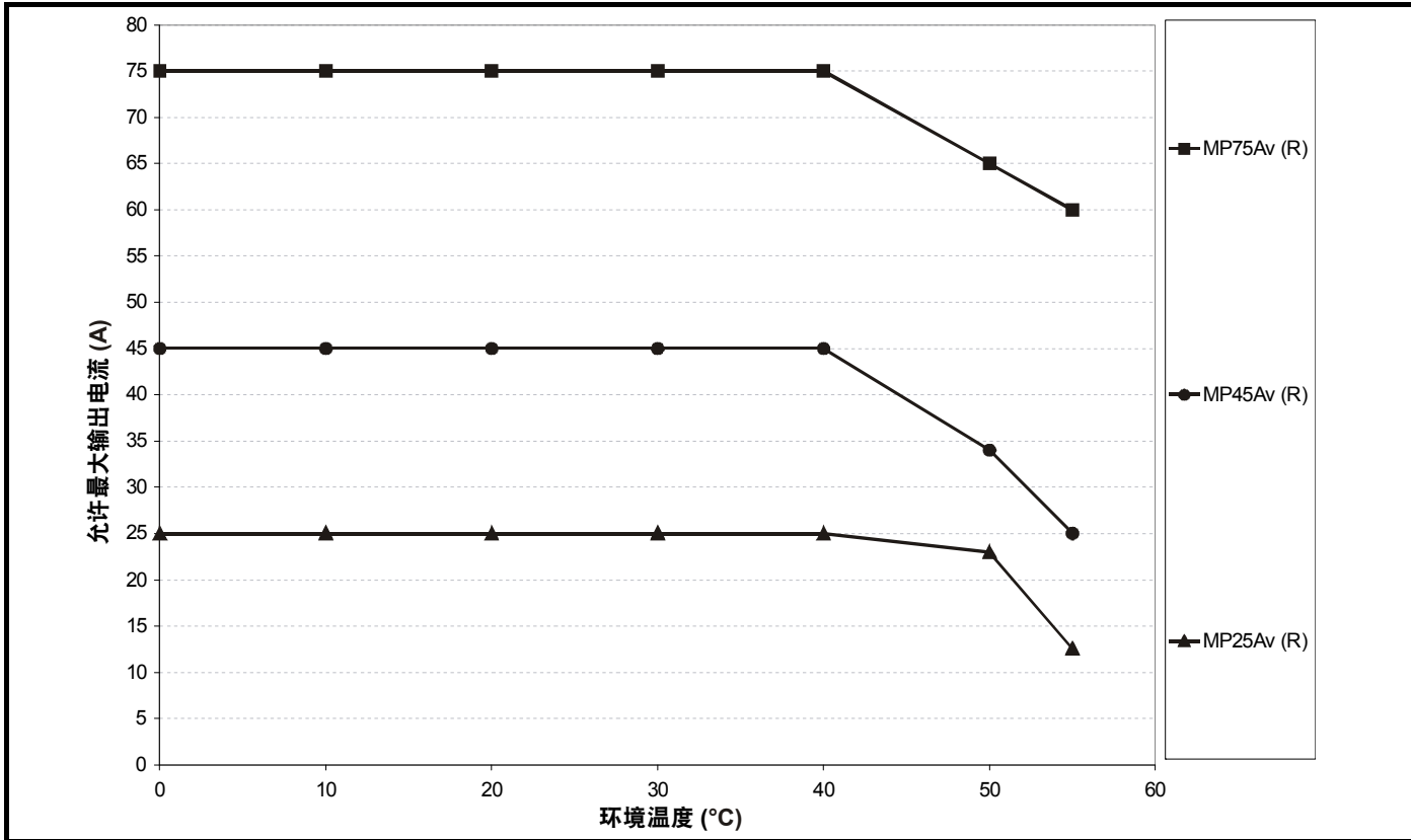
图 12-3 超出运行环境温度之外的尺寸 1B Mentor MP 的降额
