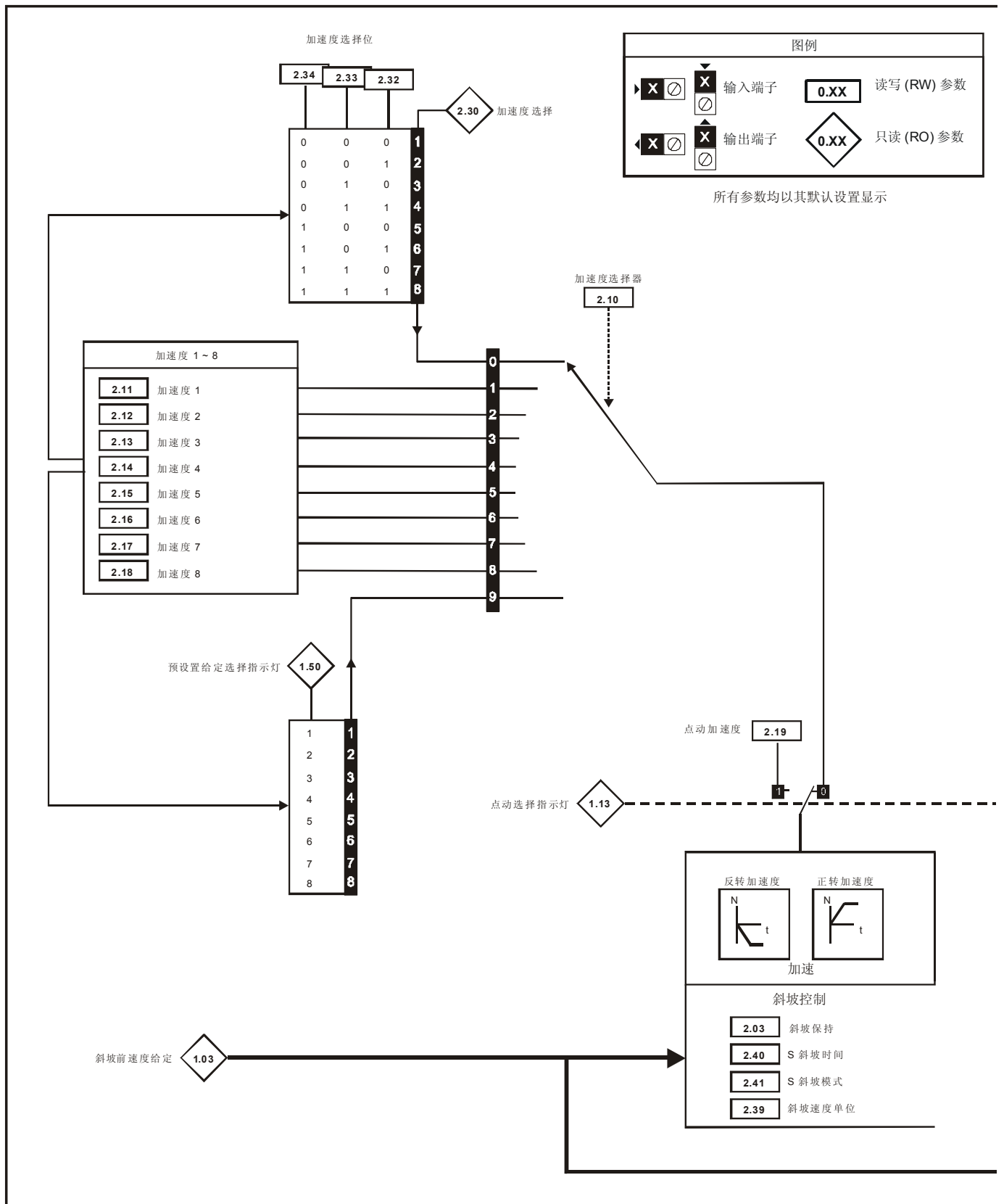
图 11-2 菜单 2 逻辑图
