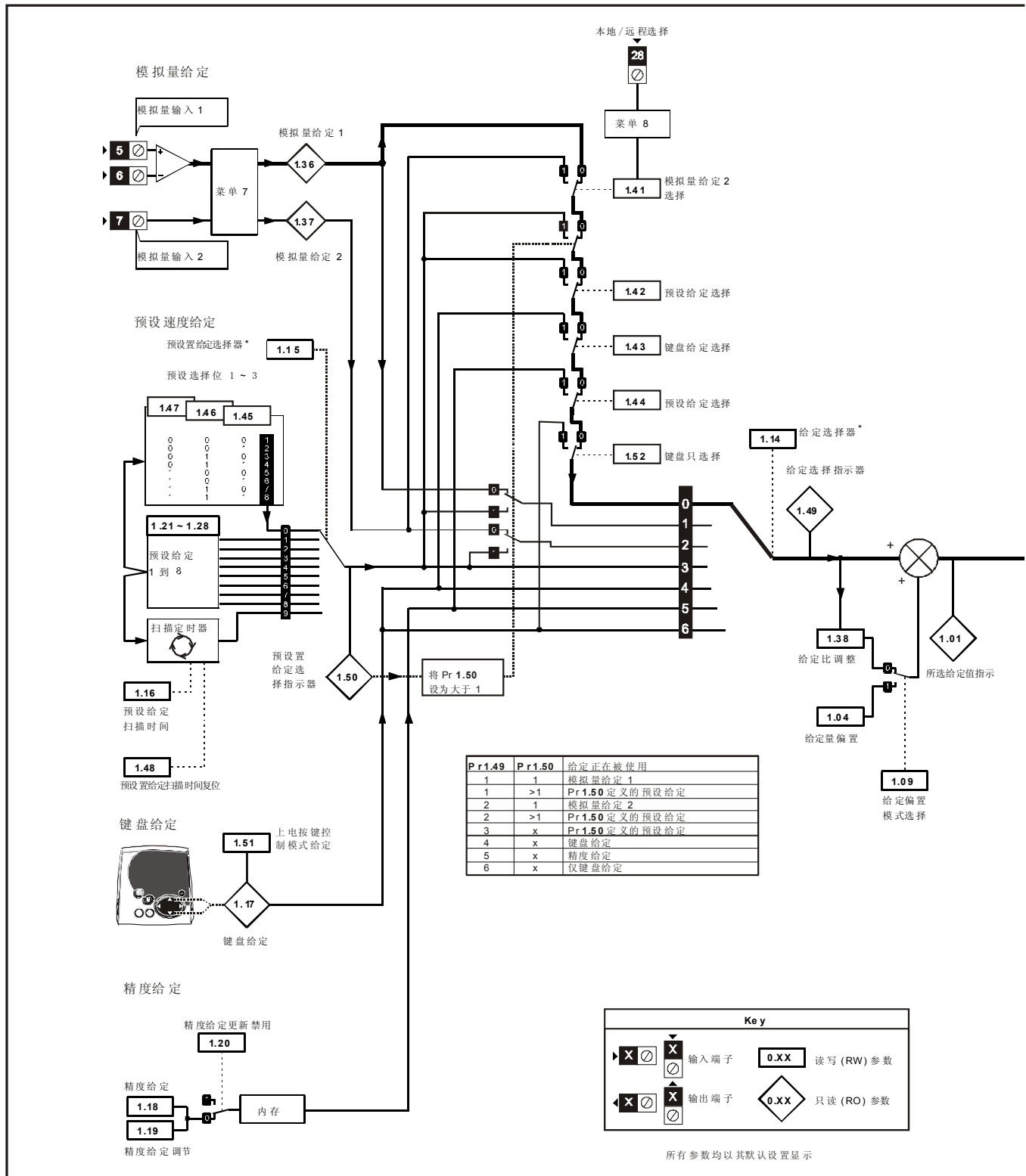
图 11-1 菜单 1 逻辑图
