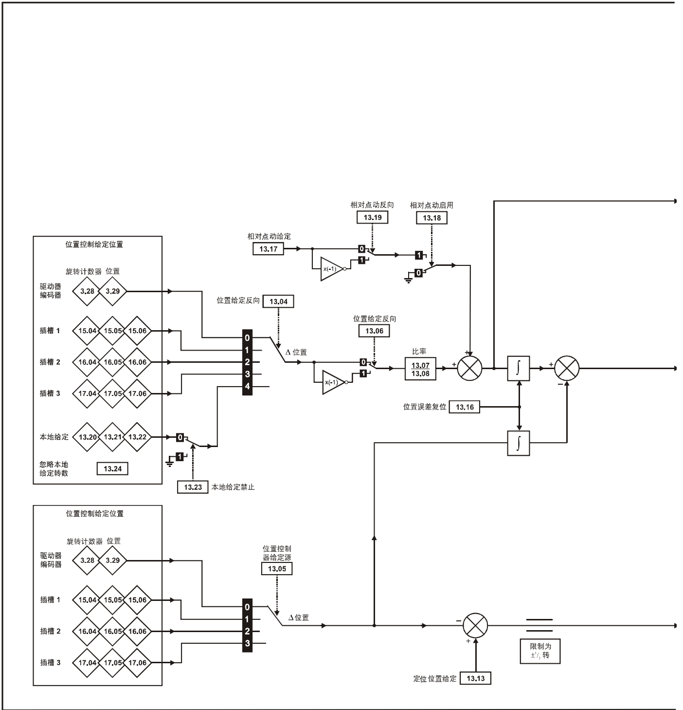
图 11-18 菜单 13 逻辑图
