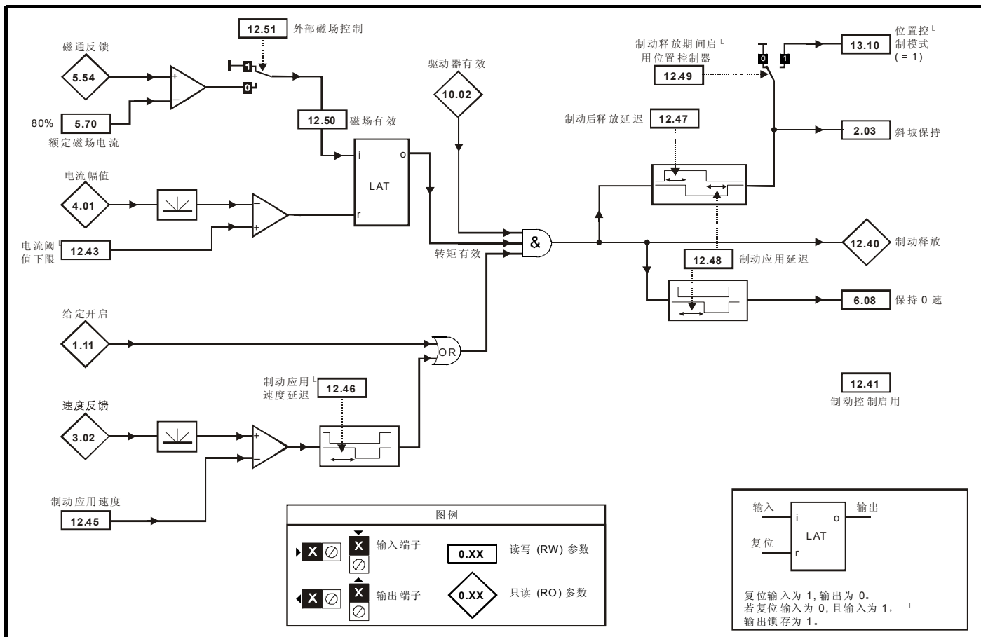
图 11-17 制动程序
