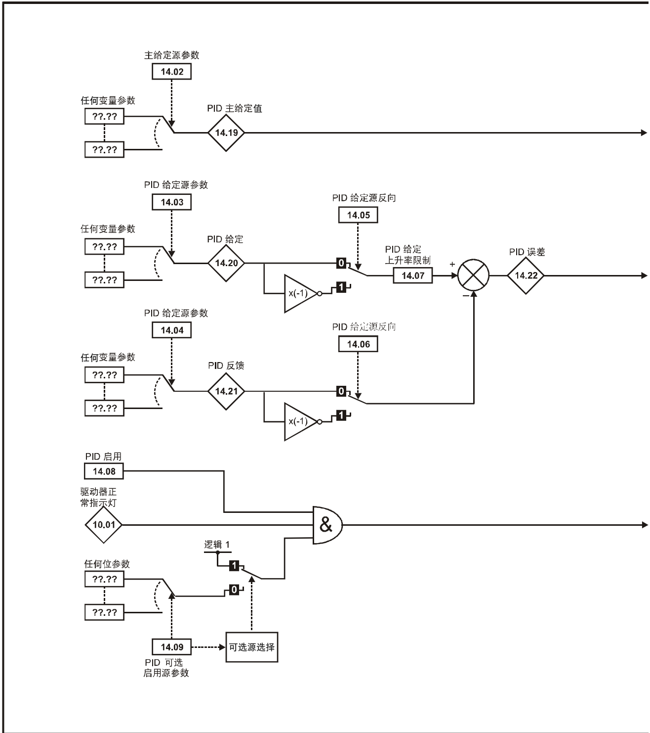
图 11-19 菜单 14 逻辑图
